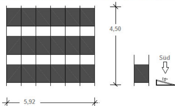
Flachdach Süd-Belegung 3 Reihen a. 6 Module
