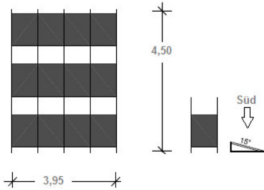
Flachdach Süd-Belegung 3 Reihen a. 4 Module
