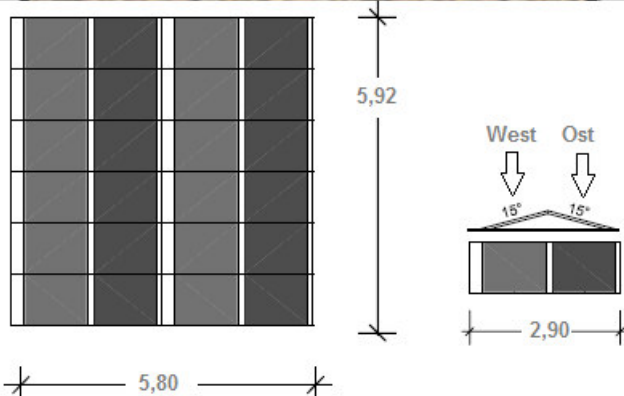
Flachdach Ost-/Westbelegung 4 Reihen a. 6 Module
